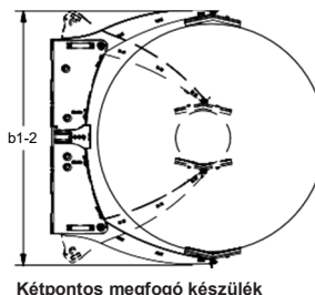
Kétpontos megfogó készülék
